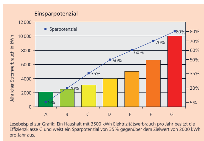
Effizienzklassen und Einsparpotenzial beim Stromverbrauch in Haushalten. Quelle: S.A.F.E.
